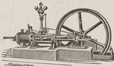
Dampfmaschine mit Schiebersteuerung.
