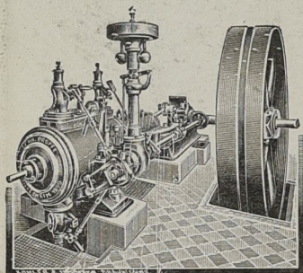
Dampfmaschine m. Ventilsteuerung.
