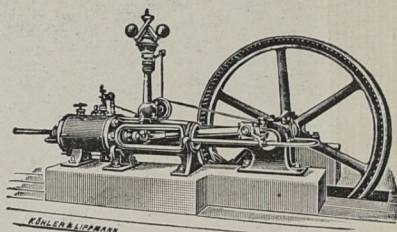
Dampfmaschine mit Schiebersteuerung.
