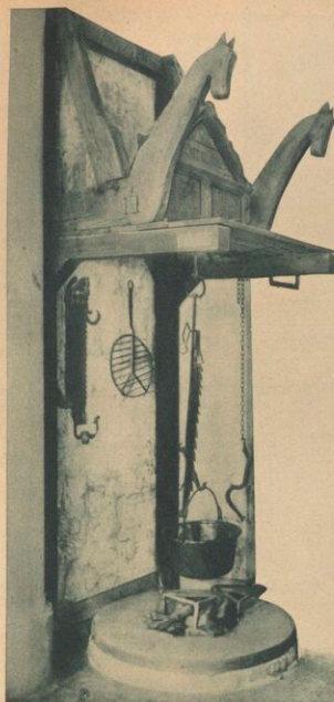
Altentümlicher Herd aus dem Jahre 1677 mit hölzernen Schutzdach, dem sogen. Rehm, darauf zwei rohgeschnitzte Pferdeköpfe
