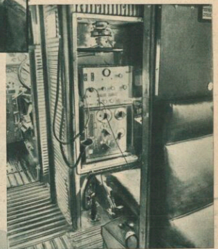
Rechts: Funkanlage in der Junkers G 31
