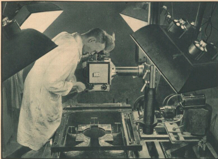
Der Apparat zur Aufnahme von Stromlinienbildern
