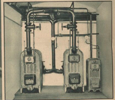
Links: Gasheizkessel-Anlage Ing. Rich. Volle, Hannover Mitte: Etagen-Heizkessel Heizungs-Seegers, Hannover Unten: Kesselanlage einer Warmwasserheizung Ing. Ludw. Keese, Hannover
